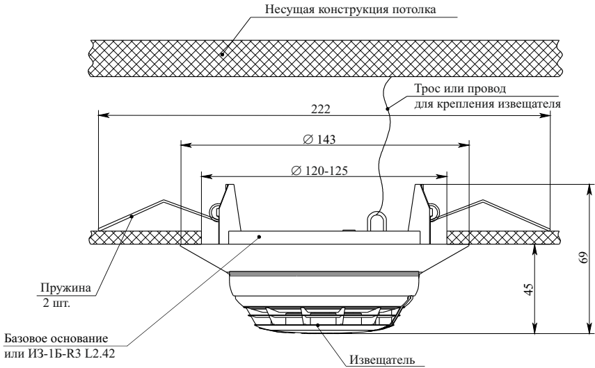
Рисунок А.2 – Установка извещателя на подвесном потолке с базовыми основаниями W2.02, W2.03 или ИЗ-1Б-Р3 L2.42
