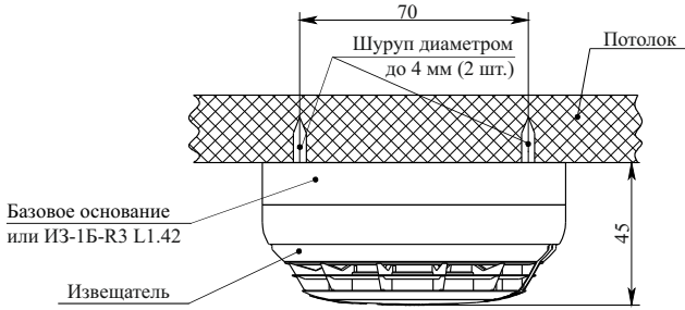
Рисунок А.1 – Установка извещателя на потолке с базовыми основаниями W1.02, W1.03 или ИЗ-1Б-Р3 L1.42
